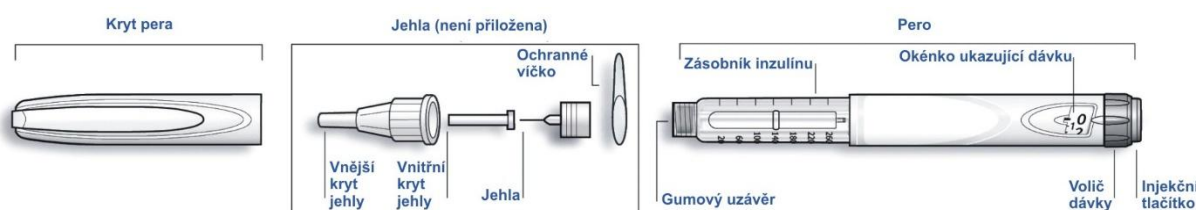
Schematický náčrt pera
