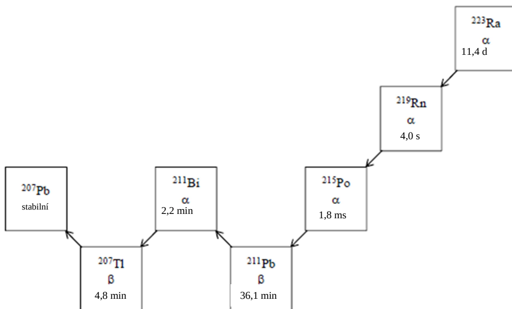
Obrázek 1: Řetězec rozpadu radia-(223Ra) s fyzikálními poločasy a způsobem rozpadu
