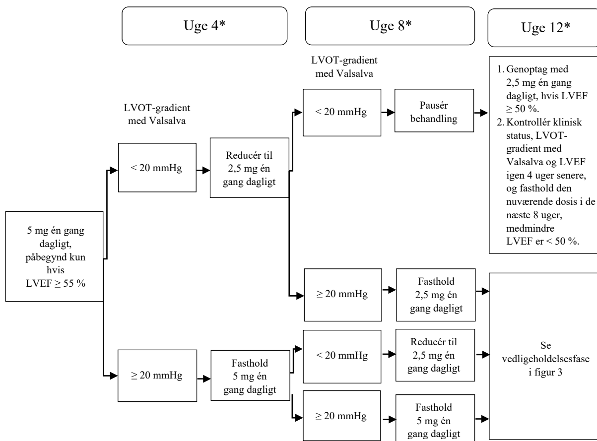
Figur 2: Påbegyndelse af behandlingen ved CYP2C19-fænotype, der er en intermediær, normal, hurtig og ultrahurtig metabolisator
