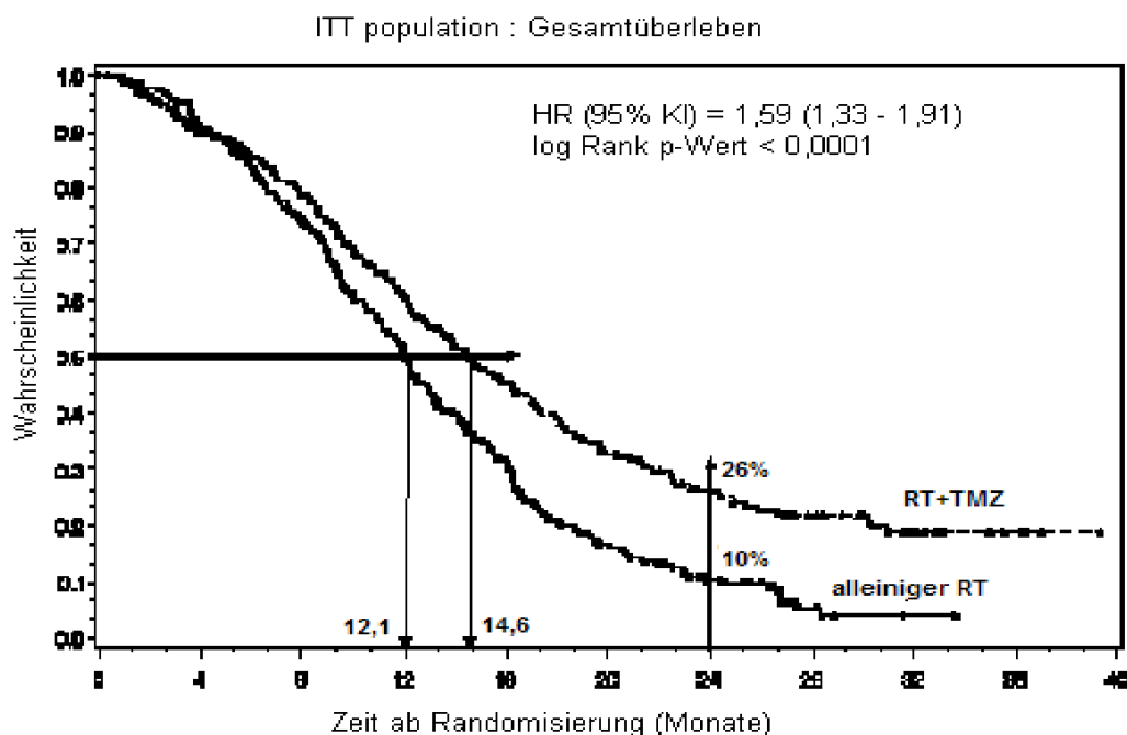
Abb. 1: Kaplan-Meier-Kurven für das Gesamtüberleben (Intent-to-Treat-Population)
