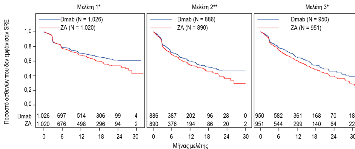
Εικόνα 1. Γραφήματα Kaplan-Meier που δείχνουν το χρόνο εμφάνισης του πρώτου σκελετικού συμβάματος κατά τη διάρκεια της μελέτης
