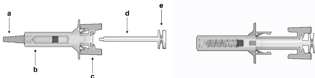
Figur 1: Sikkerhedsinjektionssprøjte: Inden brug a) Kanylehætte, b) Injektionssprøjte med kanylebeskytter, c) Beskyttelsesvinger til injektionssprøjte, d) Stempel, e) Stempelhoved
