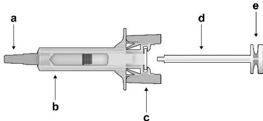
Afbeelding 1: Veiligheidsspuit: Vóór gebruik
