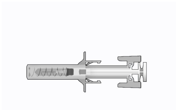
Varnostna brizga: po uporabi (Z aktiviranim mehanizmom za zaščito igle)
