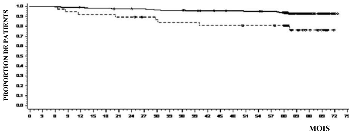
Figure 4 : Courbe de survie globale pour le dasatinib en fonction du taux de BCR-ABL ( \leq 10\% ou > 10\% ) à 3 mois - étude de Phase 3 chez des patients atteints de LMC en phase chronique nouvellement diagnostiquée
