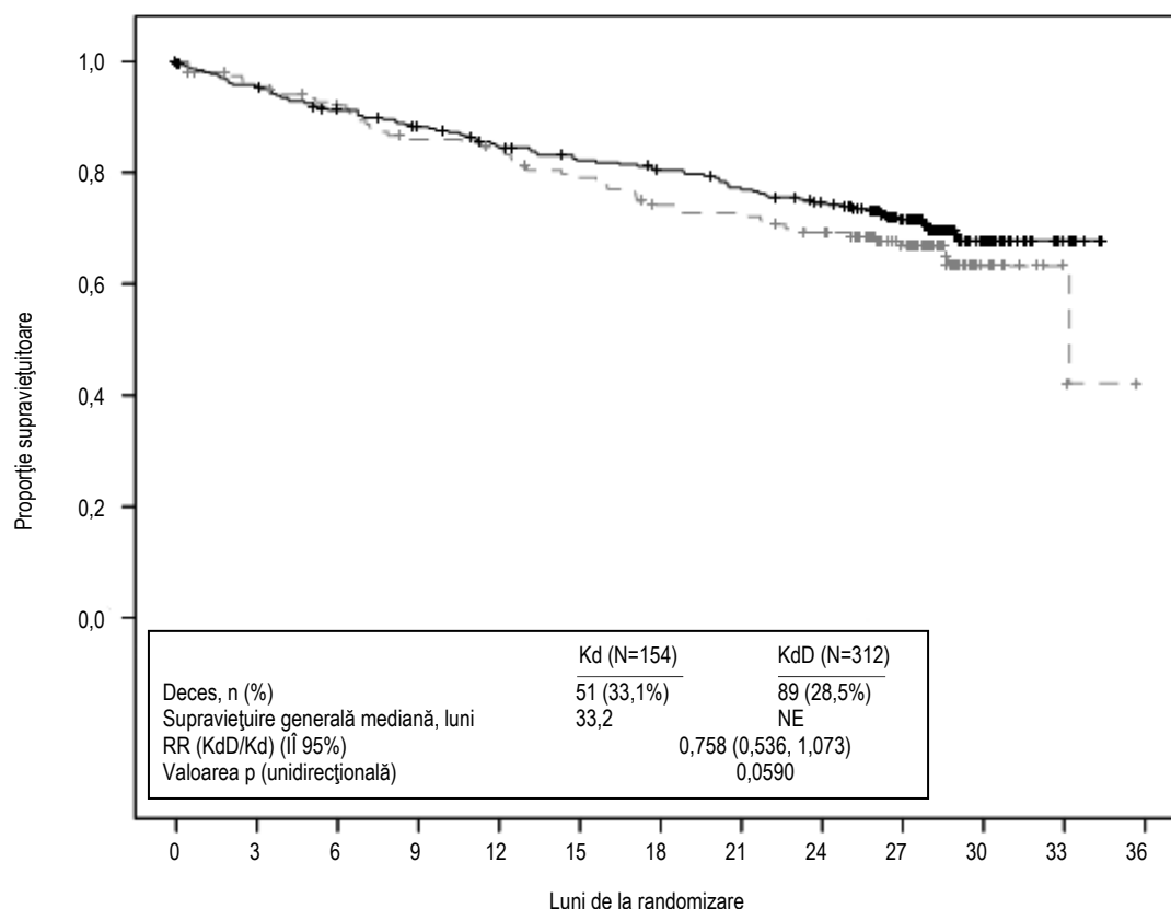
Figura 6. Curbele Kaplan-Meier corespunzătoare supraviețuirii generale în studiul 20160275
