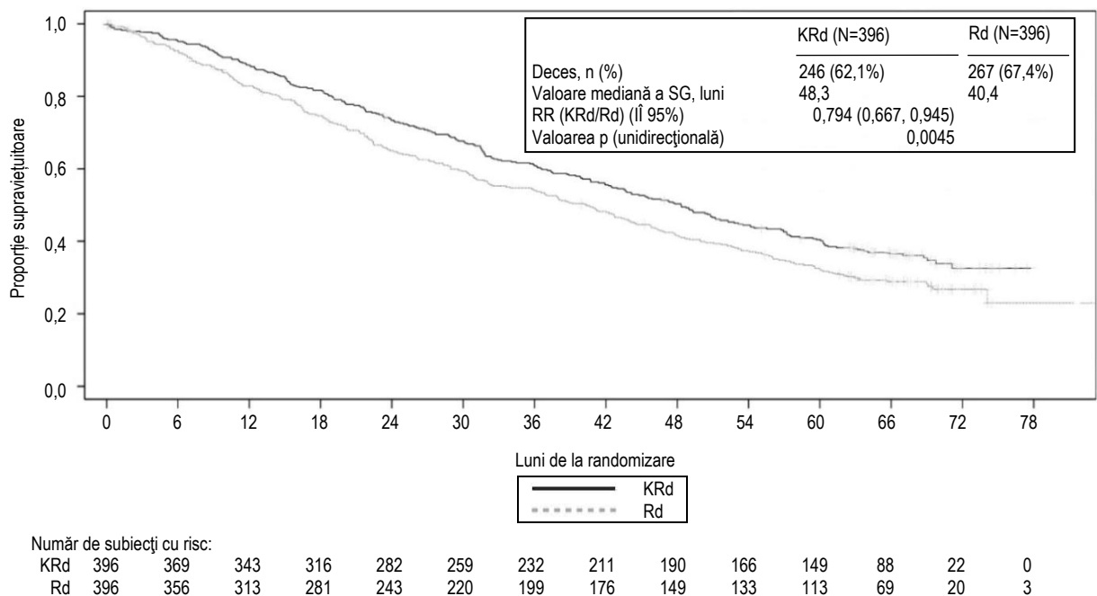
Figura 2. Curba Kaplan-Meier pentru supraviețuirea globală în mielomul multiplu recidivat a
