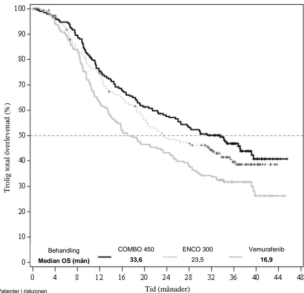
Figur 2 Studie CMEK162B2301, Part 1: Kaplan-Meier plot över interimresultat för total överlevnad (slutdatum: 7 November 2017)
