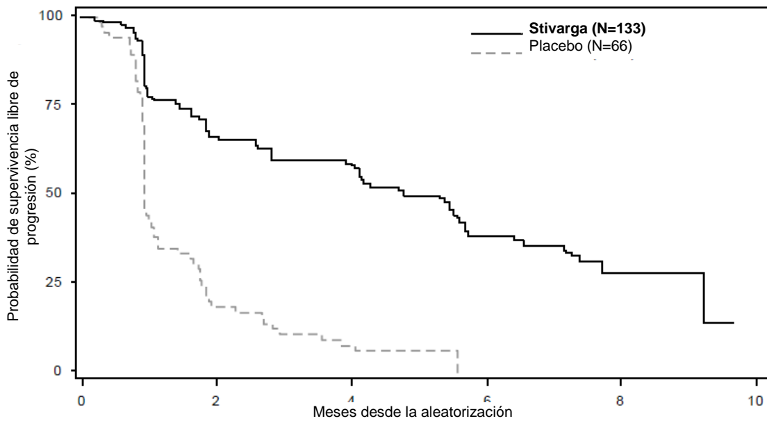
Figura 2: Curvas de Kaplan-Meier de la SLP
