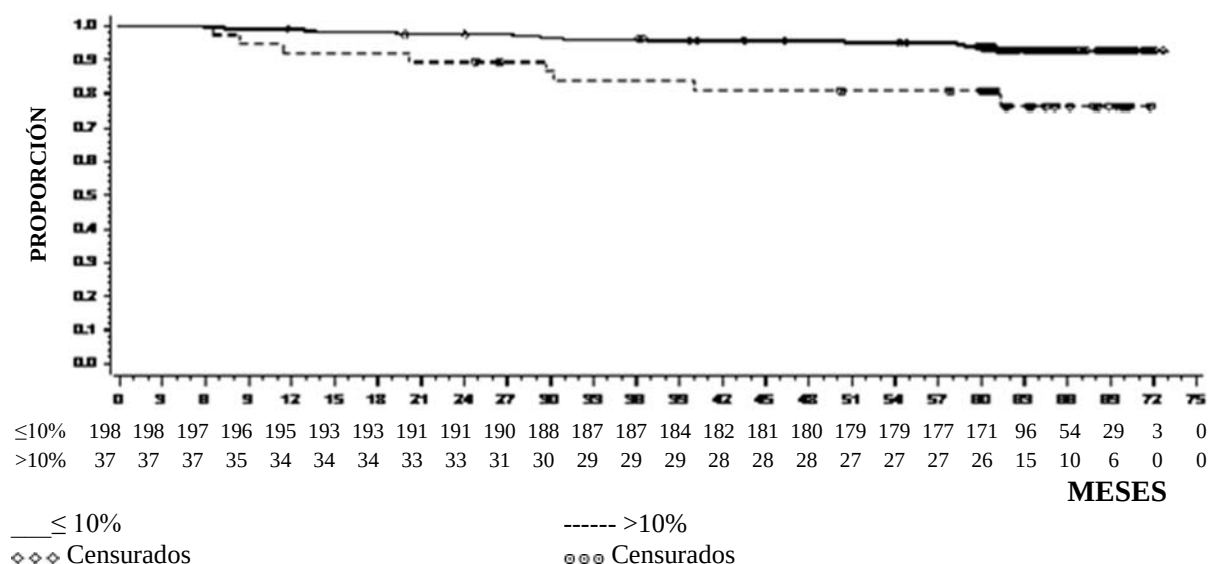
Figura 4: Curva de supervivencia global para dasatinib por nivel de BCR-ABL ( \leq 10\% o >10\% ) a 3 meses en un ensayo fase 3 en pacientes con LMC en fase crónica de nuevo diagnóstico
