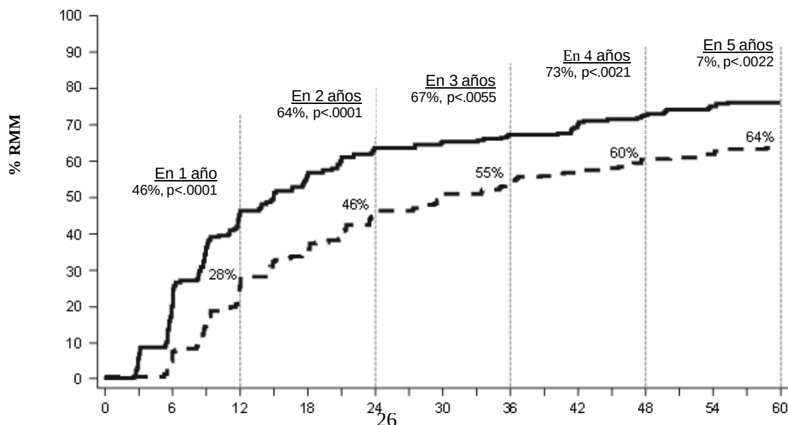
Figura 2: Tasas de RMM en el tiempo - todos los pacientes aleatorizados en un ensayo fase 3 con LMC en fase crónica de nuevo diagnóstico
