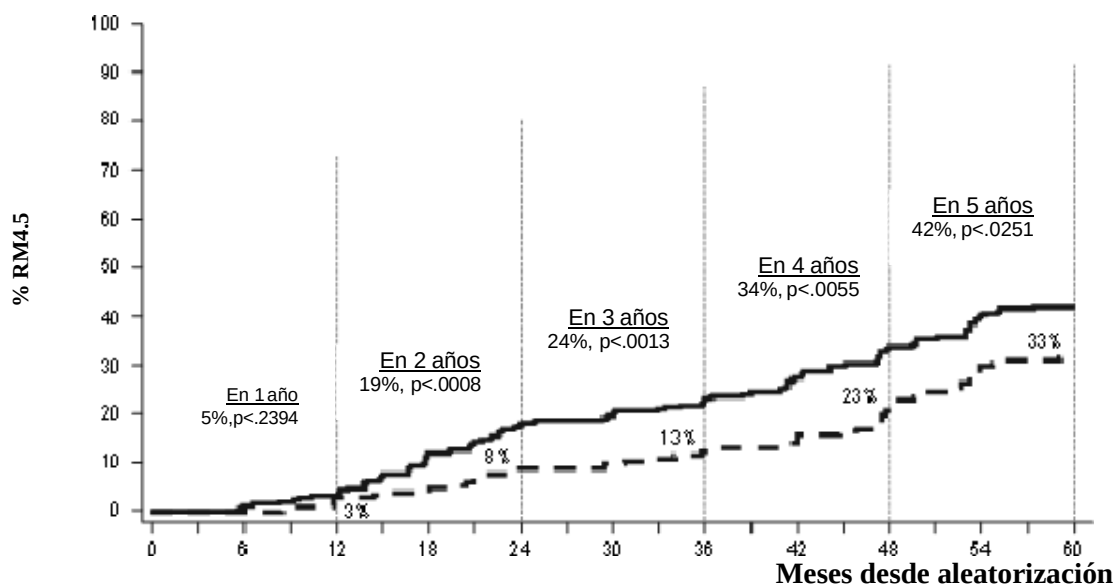
Figura 3: Tasas RM4,5 a lo largo del tiempo - todos los pacientes aleatorizados en un ensayo fase 3 con LMC en fase crónica de nuevo diagnóstico
