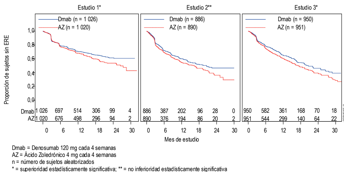
Figura 1. Gráficos de Kaplan-Meier del tiempo hasta el primer ERE durante el estudio
