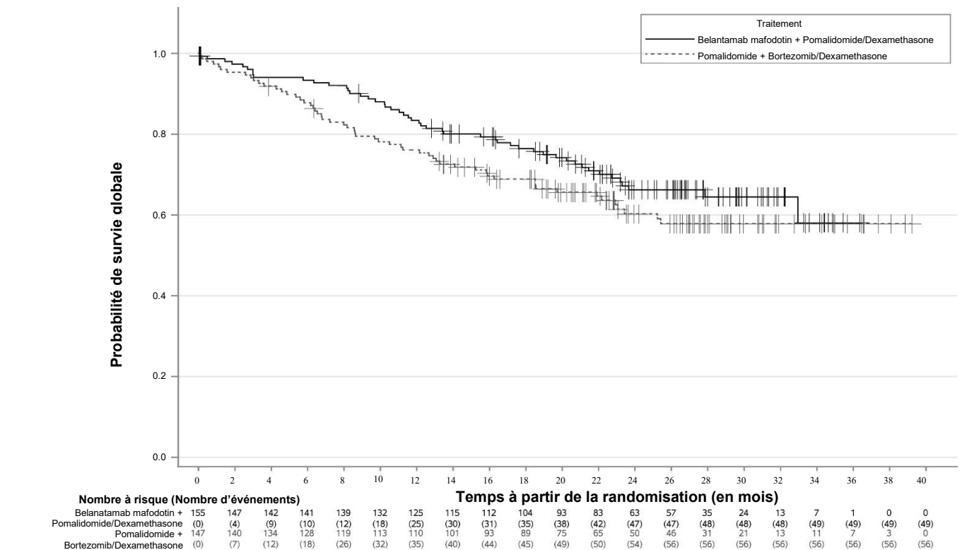
Figure 4 : Courbe de Kaplan-Meier de survie globale dans DREAMM-8
