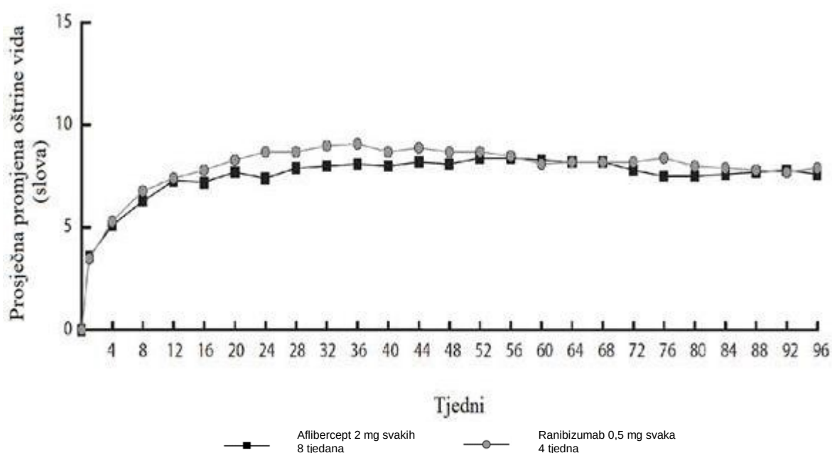
Slika 1. Srednja vrijednost promjene oštrine vida od početne vrijednosti do 96. tjedna za kombinirane podatke iz ispitivanja VIEW1 i VIEW2
