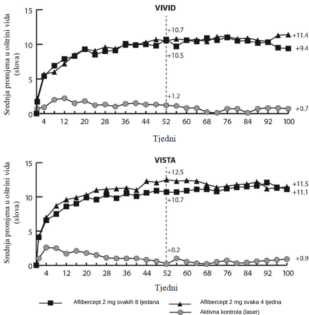
Slika 4: Srednja vrijednost promjene BCVA mjereno pomoću ETDRS slovnog rezultata u 100. tjednu u odnosu na početnu vrijednost u ispitivanjima VIVID DME i VISTA DME
