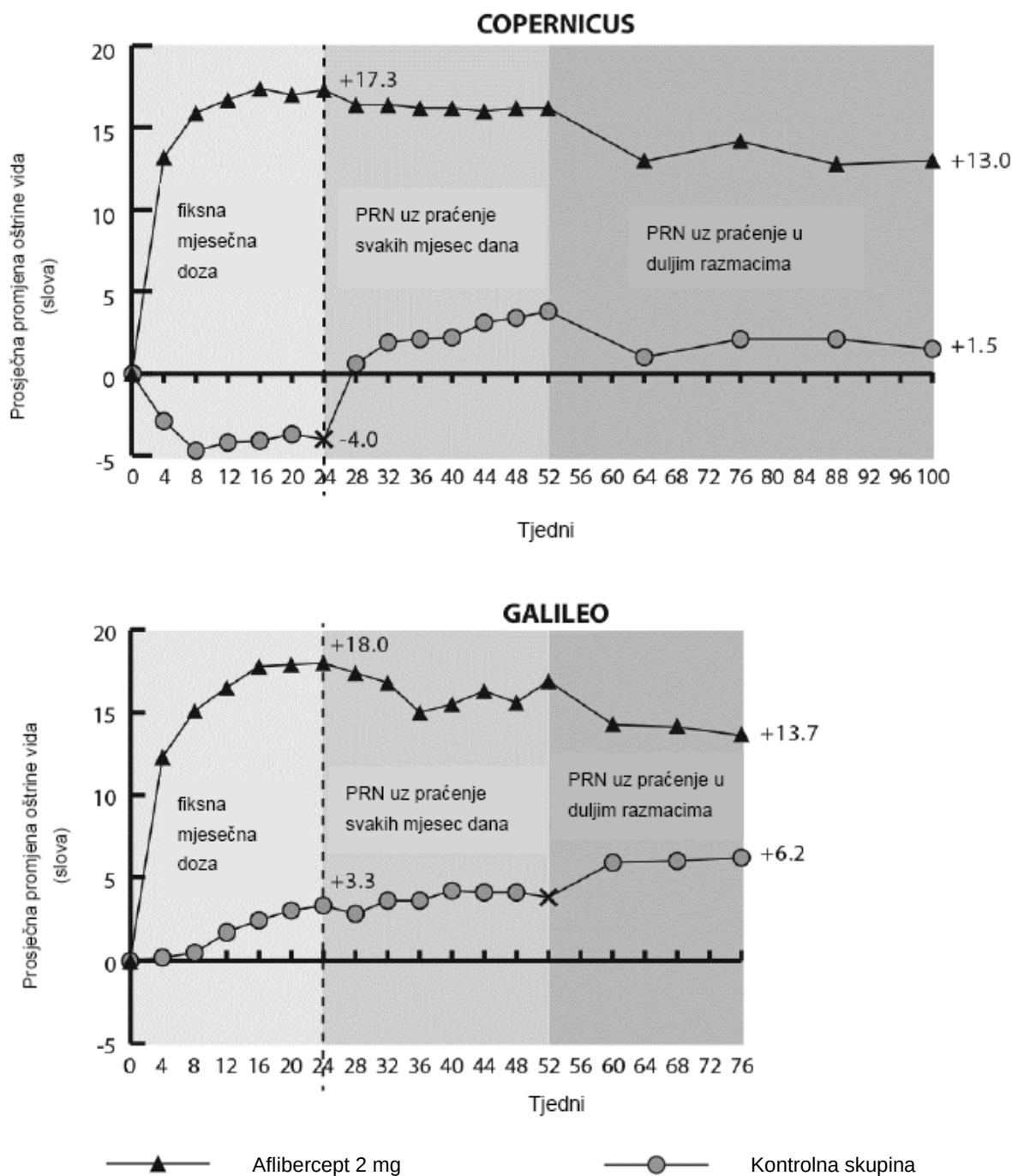
Slika 2: Srednja vrijednost promjene od početne vrijednosti do 76./100. tjedna u oštrini vida po terapijskim skupinama u ispitivanju COPERNICUS i ispitivanju GALILEO (analiza svih podataka)
