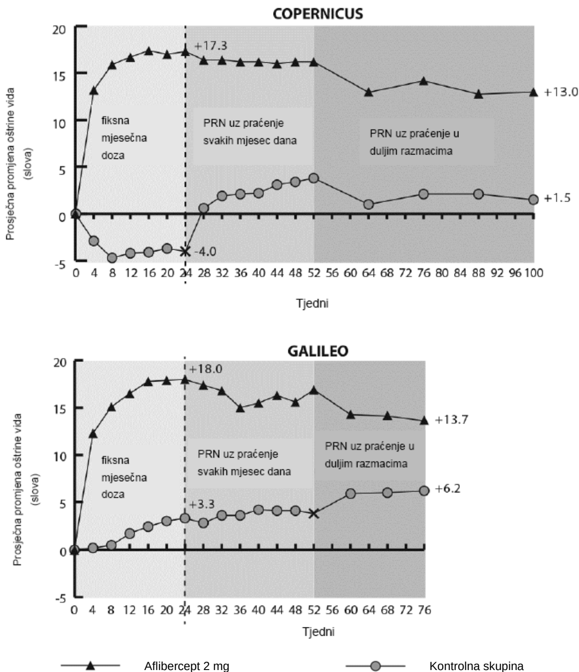
Slika 2: Srednja vrijednost promjene od početne vrijednosti do 76./100. tjedna u oštini vida po terapijskim skupinama u ispitivanju COPERNICUS i ispitivanju GALILEO (analiza svih podataka)
