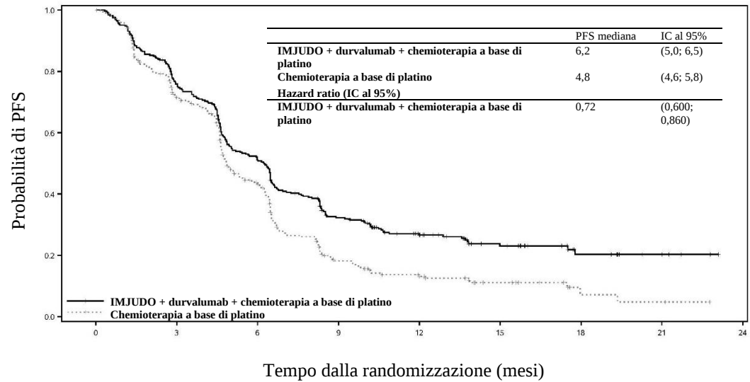
Figura 3. Curva di Kaplan-Meier della PFS
