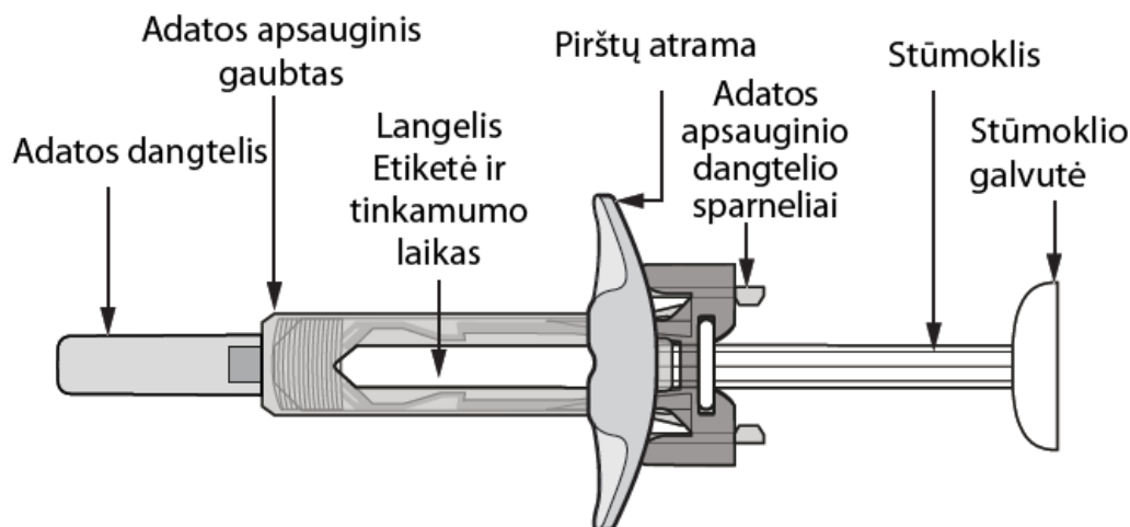
A pav. Hefiya užpildytas švirkštas su adatos apsauginiu gaubtu ir pirštų atrama
