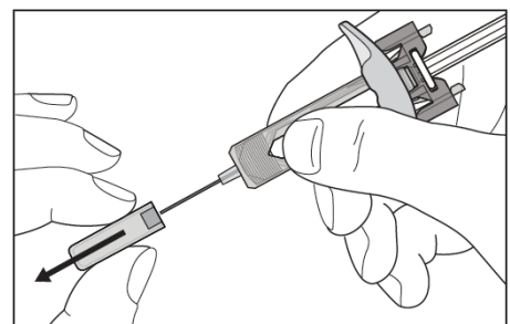
G pav. Nuimkite adatos dangtelį
