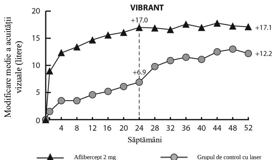
Figura 3: Studiul clinic VIBRANT - Modificarea medie a AVOC măsurată prin scorul literelor ETDRS față de momentul inițial în săptămâna 52
