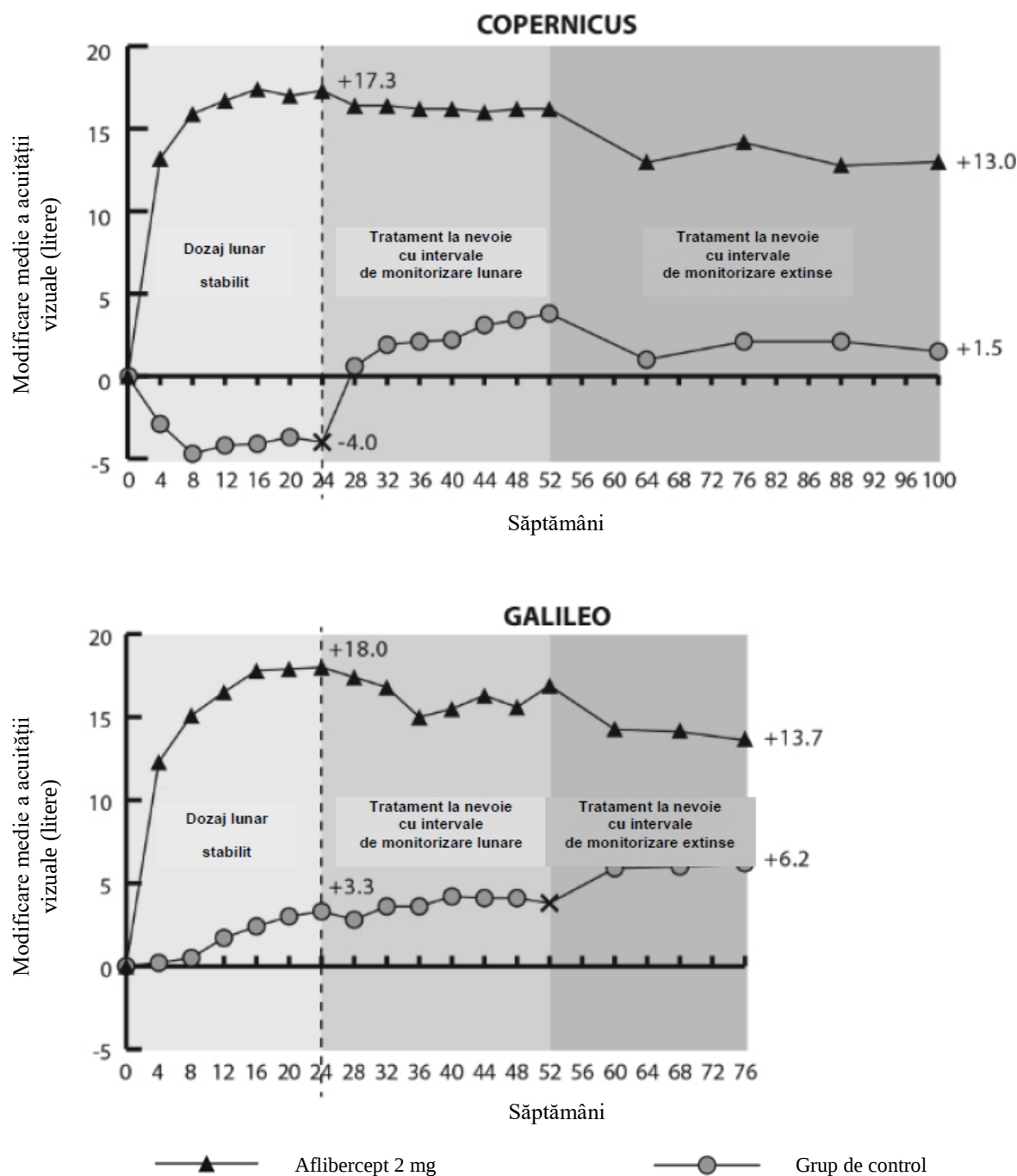
Figura 2: Modificarea medie de la momentul inițial în săptămâna 76/100 în ceea ce privește acuitatea vizuală în funcție de grupul de tratament pentru studiile COPERNICUS și GALILEO (Set complet de analiză)
