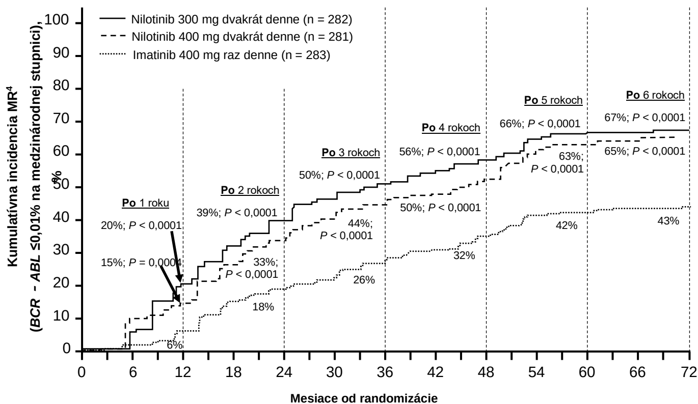
Obrázok 2 Kumulatívna incidencia molekulovej odpovede \leq 0,01\% (zníženie 4 log)
