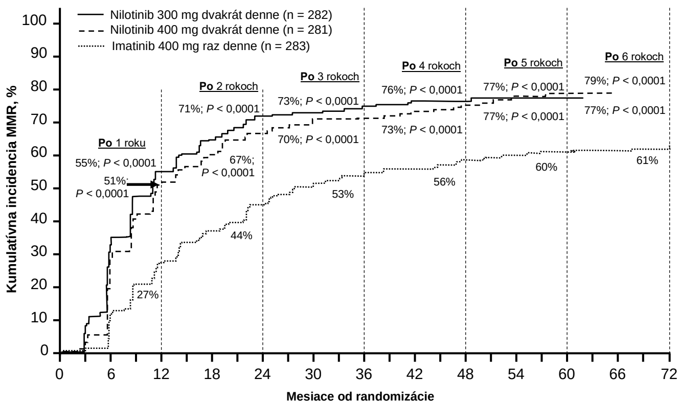
Obrázok 1 Kumulatívna incidencia MMR
