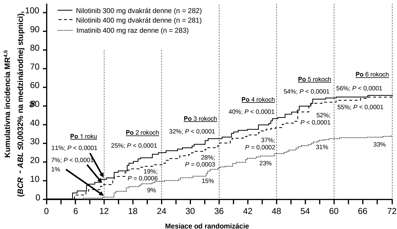
Obrázok 3 Kumulatívna incidencia molekulej odpovede \leq 0,0032\% (zniženie 4,5 log)
