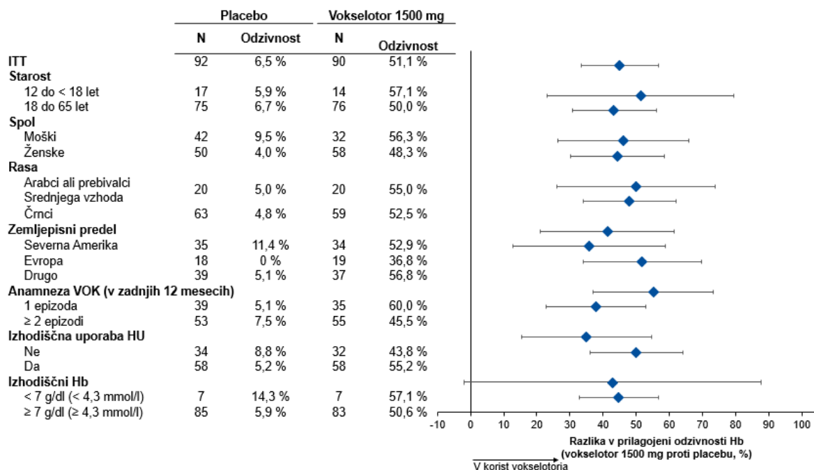
Slika 1: Odziv hemoglobina v 24. tednu po podskupinah (vokselotor 1.500 mg proti placebu) (populacija z namenom zdravljenja [intent-to-treat (ITT) population])
