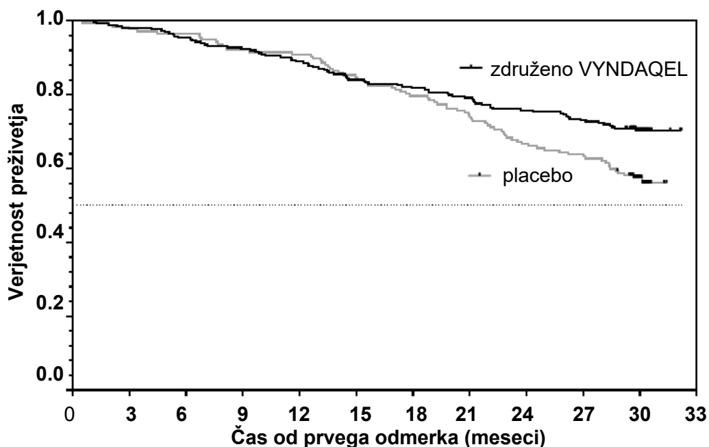
Slika 1: Umrljivost iz vseh vzrokov*
