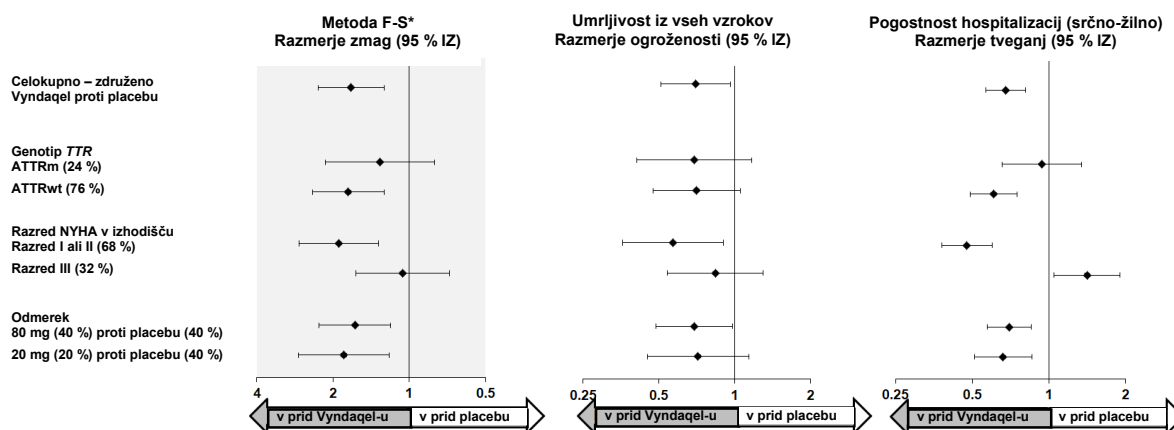
Slika 2: Rezultati po metodi F-S in komponente po podskupinah in odmerkih
