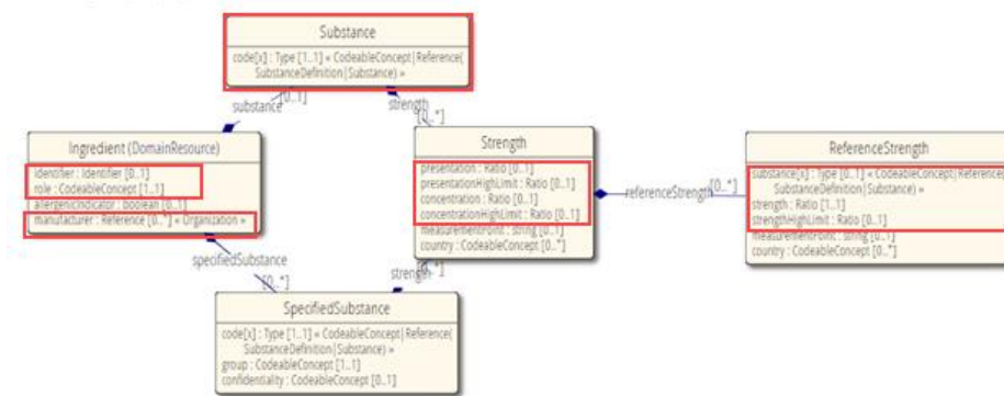
UML Diagram (Legend)
